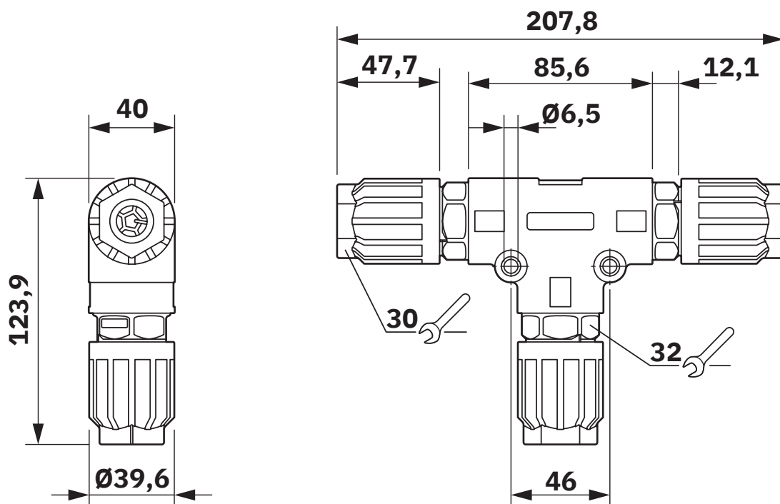
Maßzeichnung
