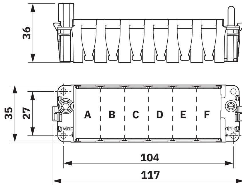
Maßzeichnung
