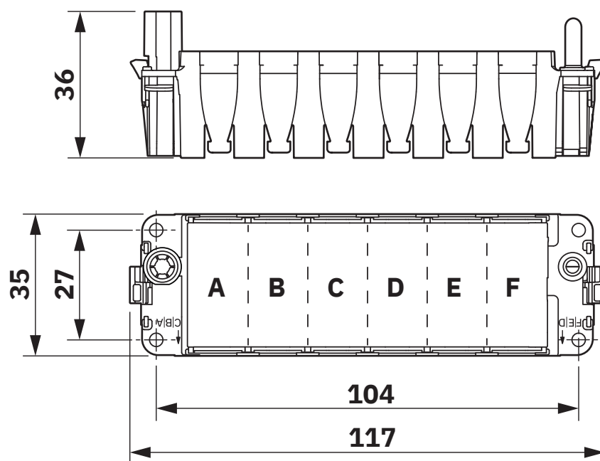
Dessin coté
