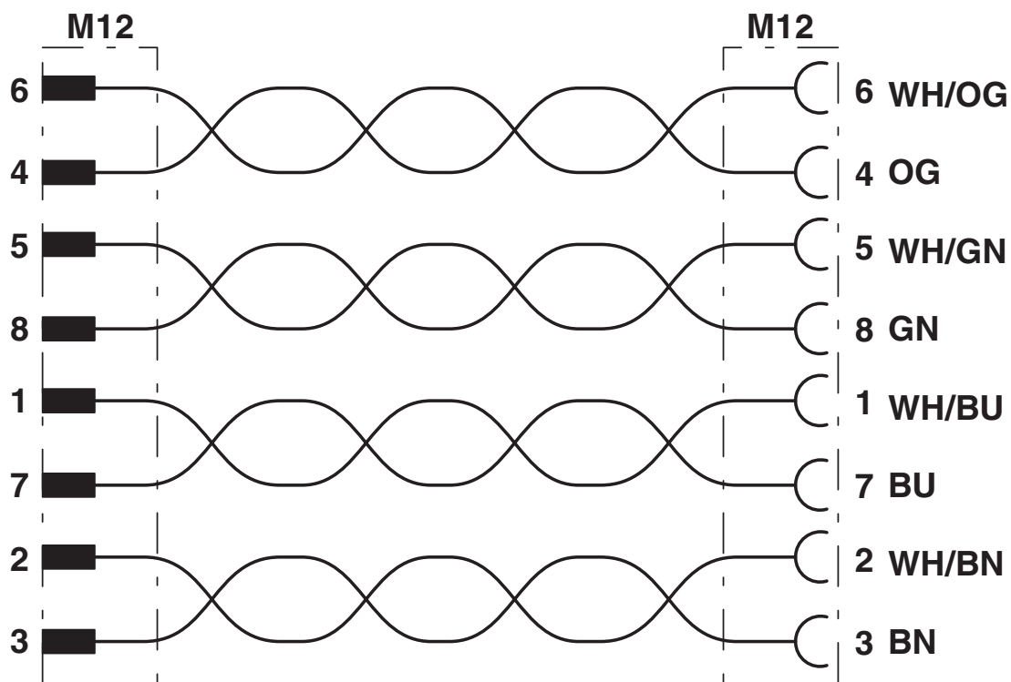
Schaltplan
