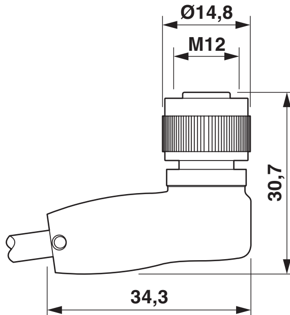
Maßzeichnung
