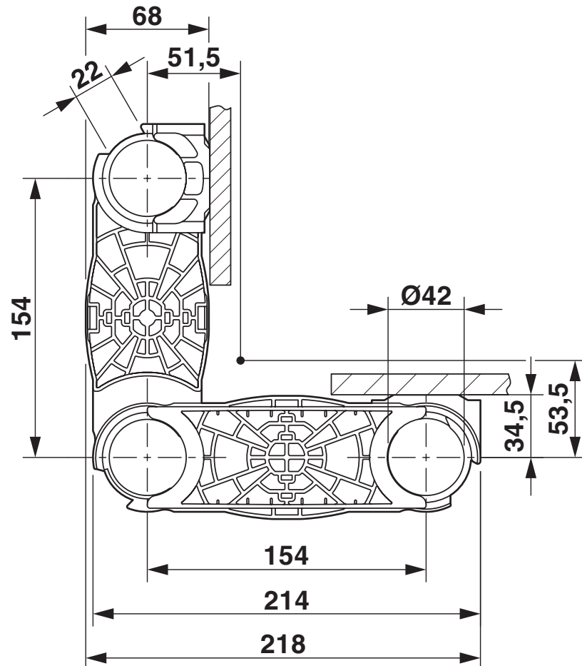
Dessin coté
