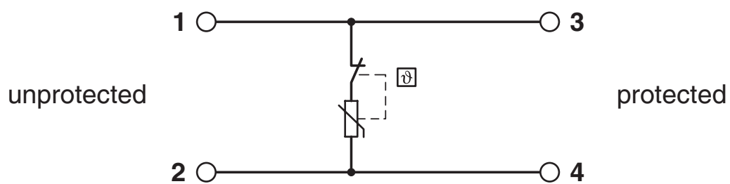
Diagrama eléctrico
