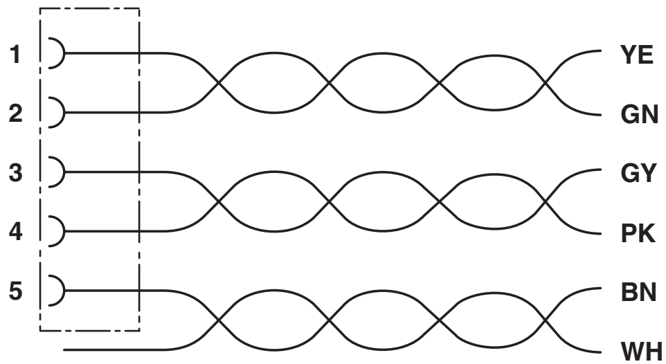
Diagrama eléctrico
