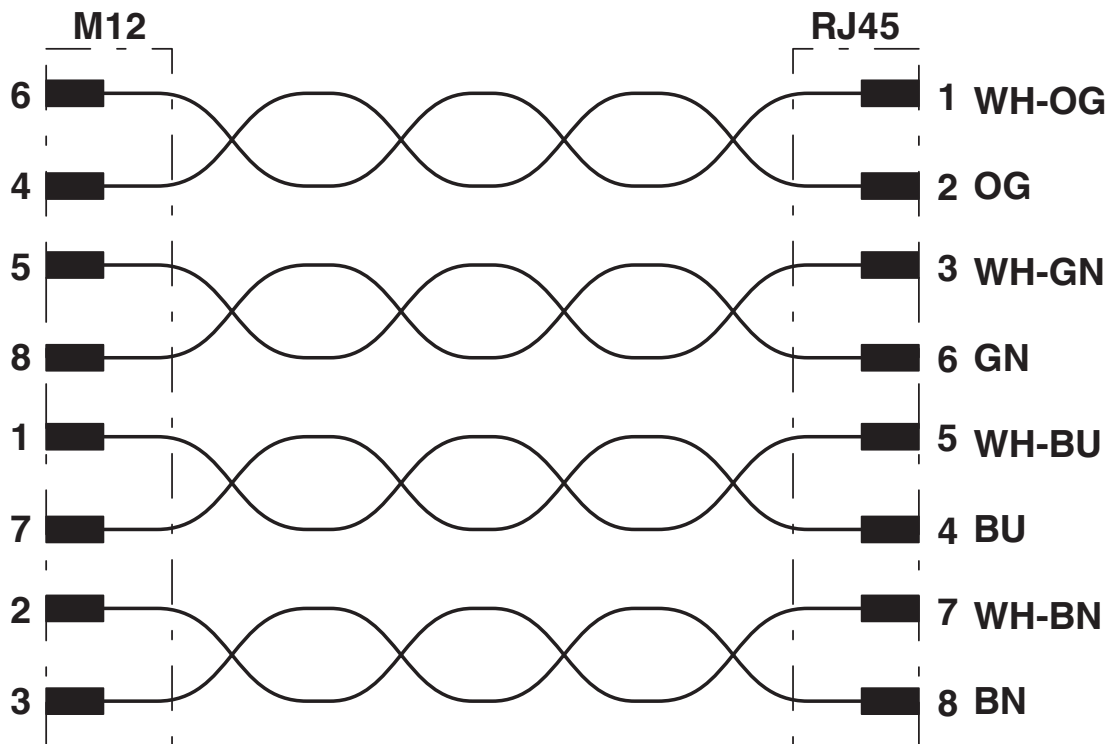
Schaltplan
