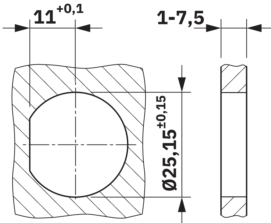
Esquema de taladros
