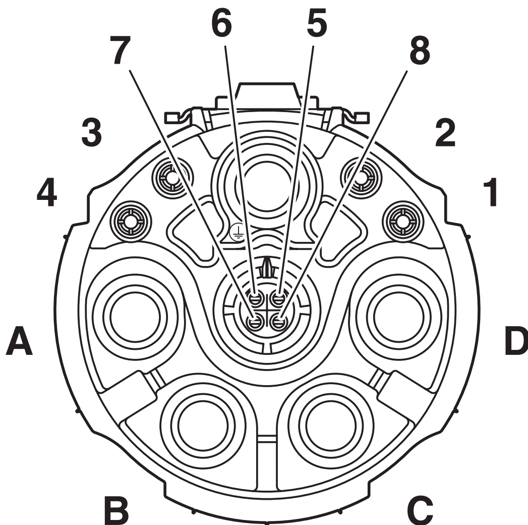
Dessin schématique
