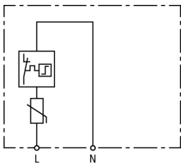
Esquema del DCOR L 1P 275
