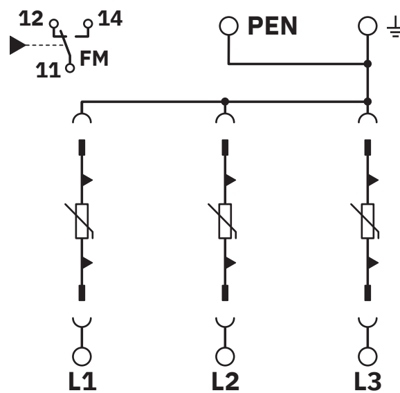
Schaltplan
