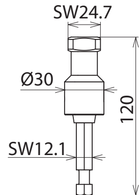
Maßbild AK SK24 SK12
