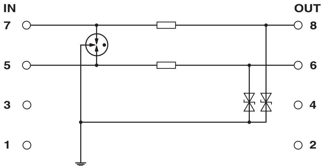
Schaltplan
