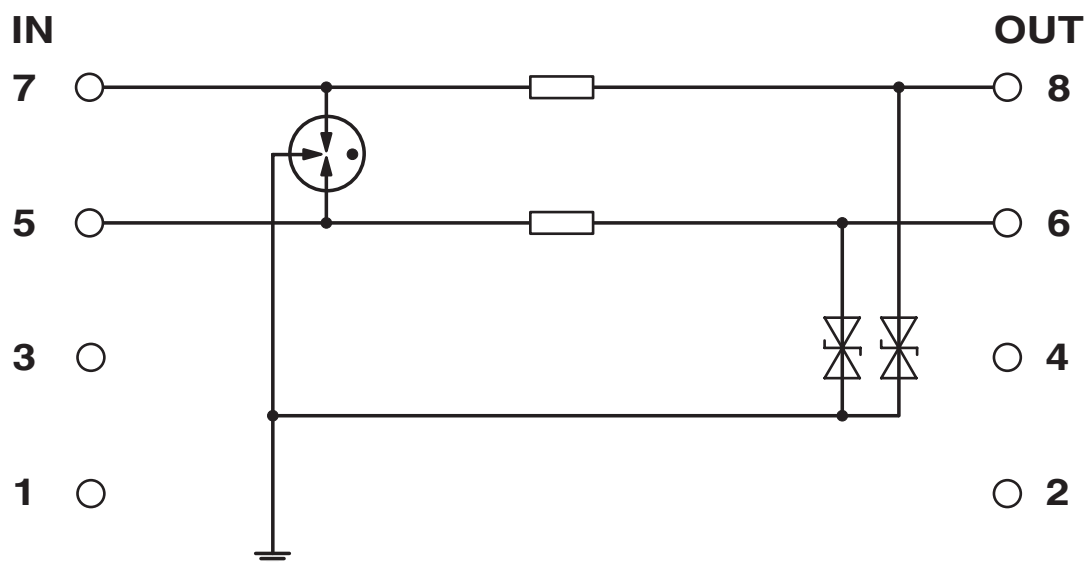
Diagrama eléctrico
