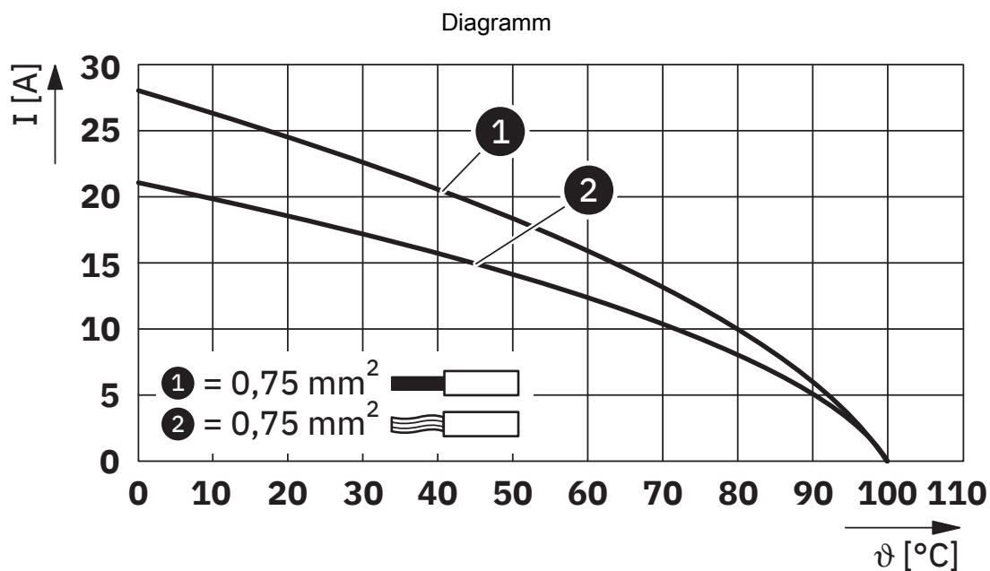
Derating-Diagramm für 0,75 mm 2
