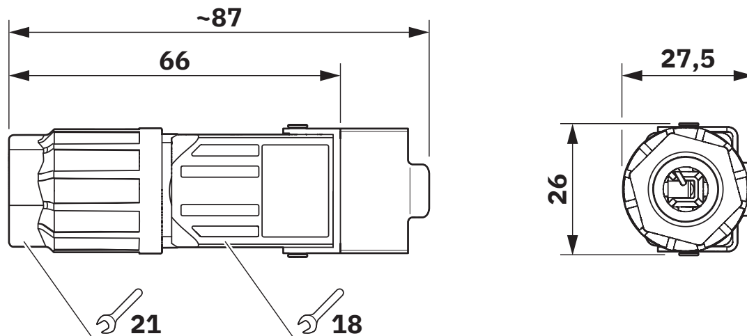
Maßzeichnung
