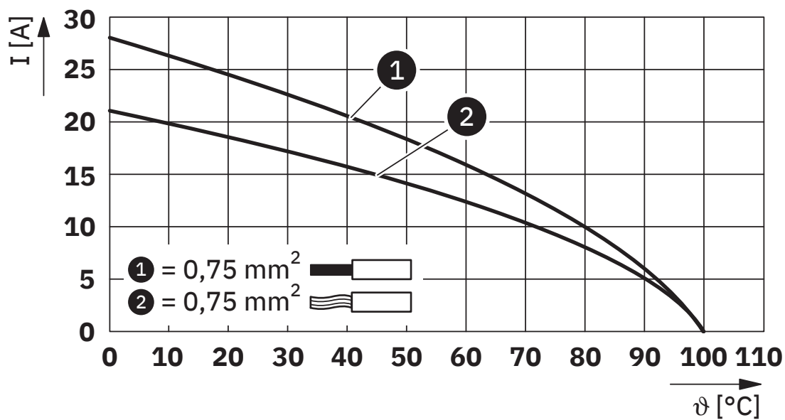
Diagrama de derating para 0,75 mm 2
