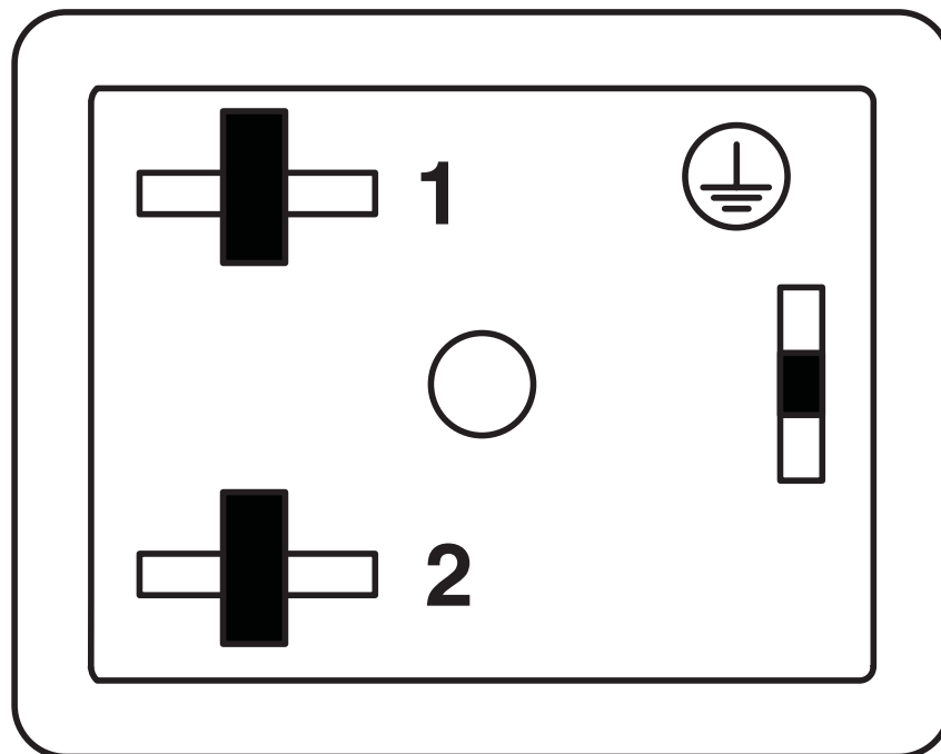
Plano esquemático
