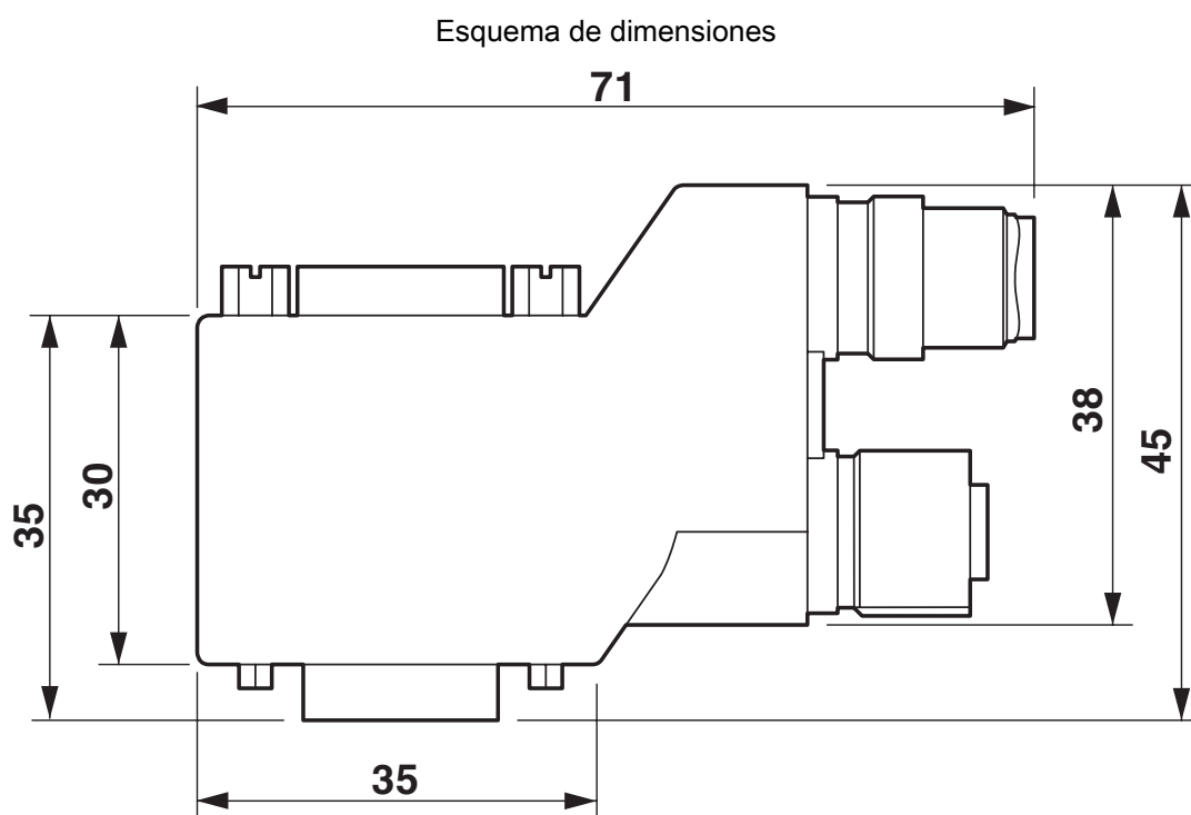
Esquema de dimensiones SUBCON-PLUS...90...M12, variante corta de 90°
