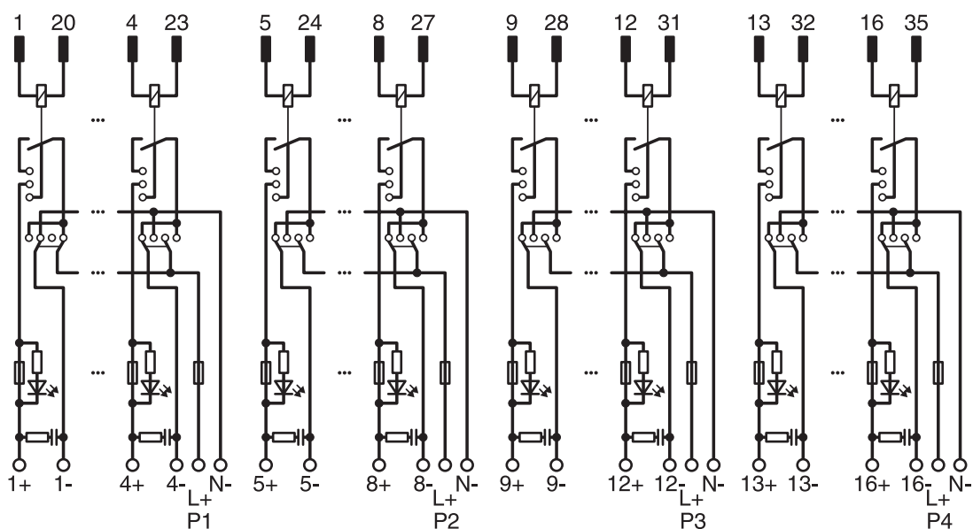
Diagrama eléctrico
