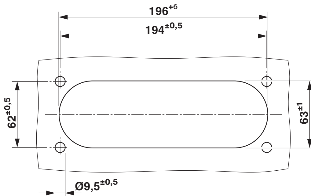
Dibujo de la sección de pared
