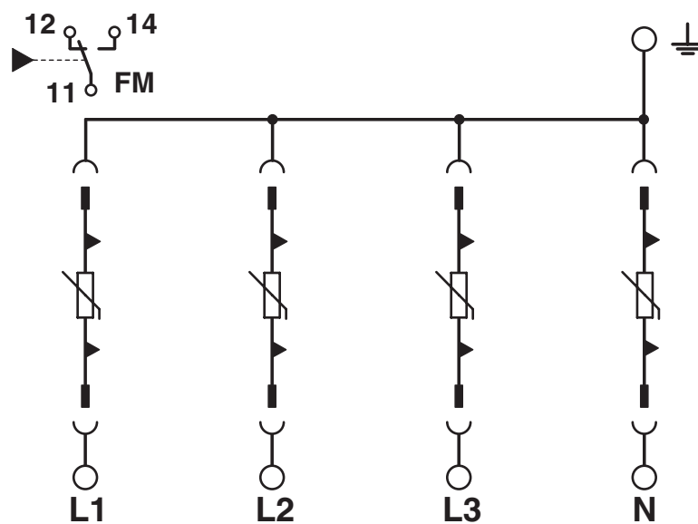
Schaltplan
