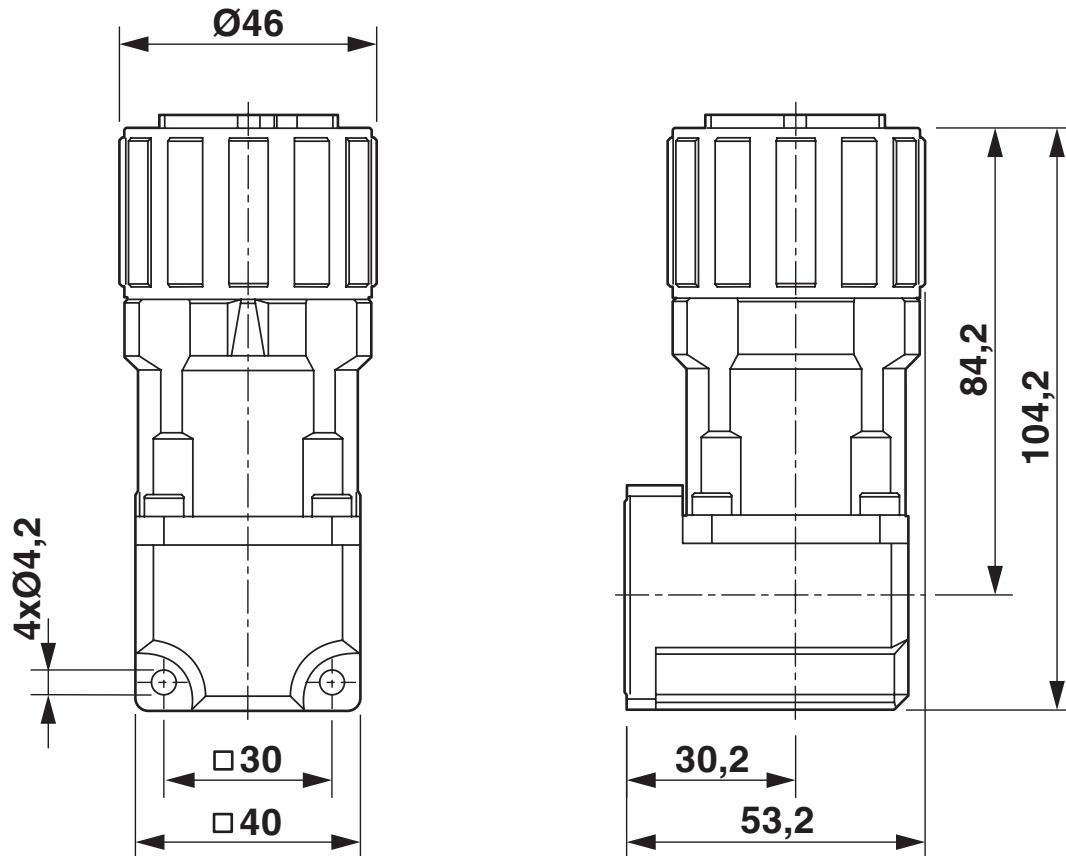
Maßzeichnung
