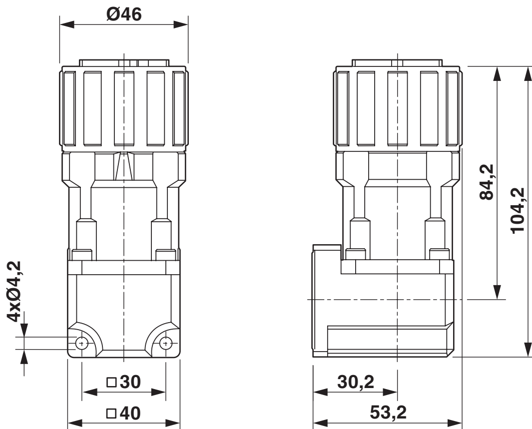
Dessin coté
