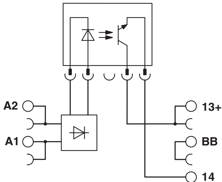
Schaltplan
