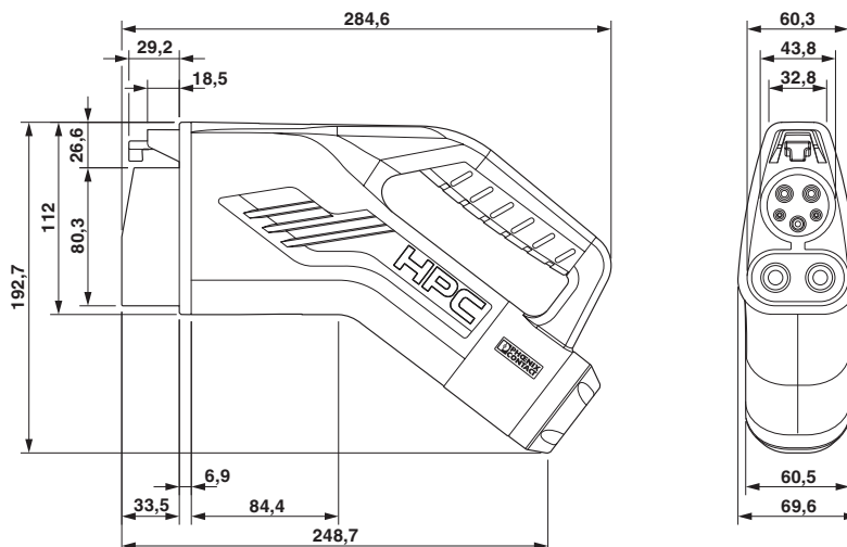
Dessin coté
