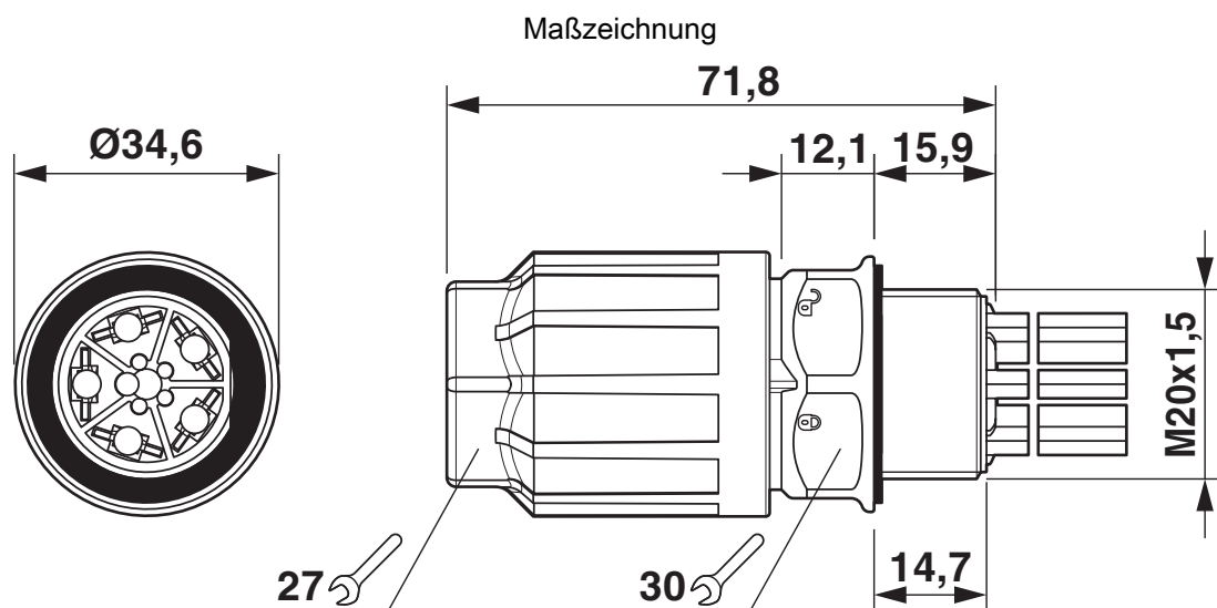
Maßzeichnung des QPD W 5x2,5 M20
