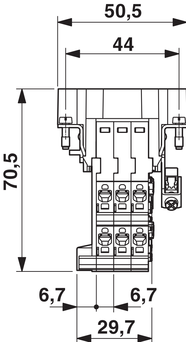
Maßzeichnung
