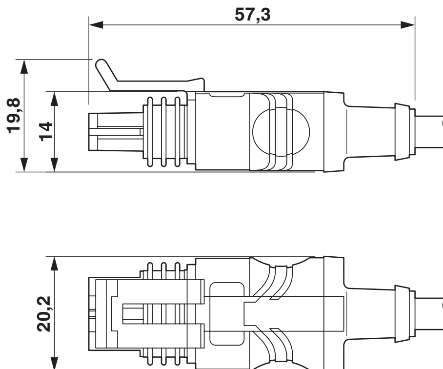
Superseal, conector hembra, vista superior y lateral
