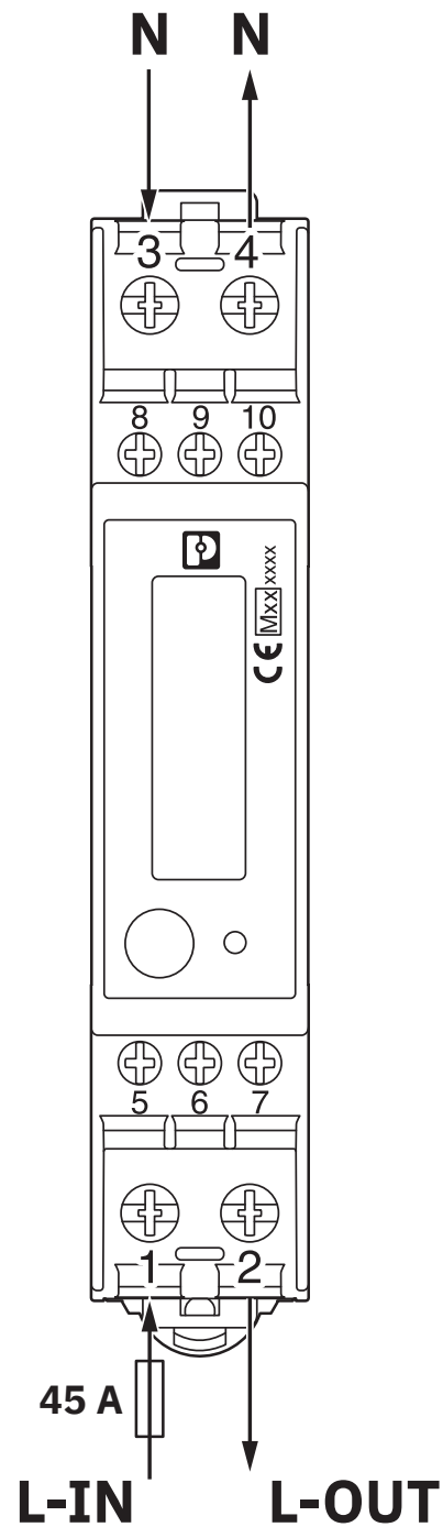
Anschlusszeichnung
