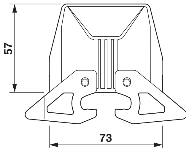
Dessin coté
