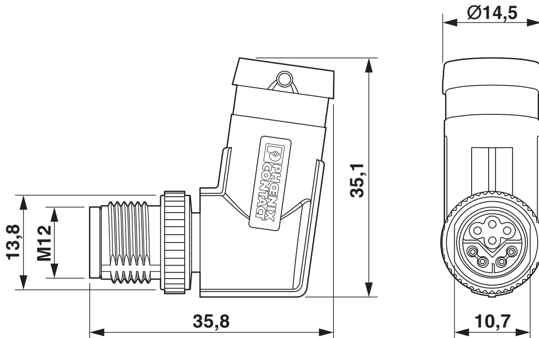
Maßzeichnung
