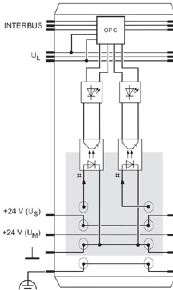
Blockschaltbild
