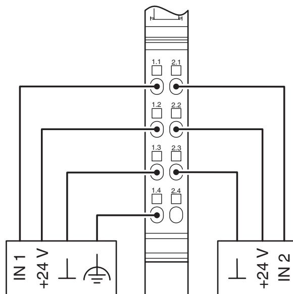
Anschlusszeichnung
