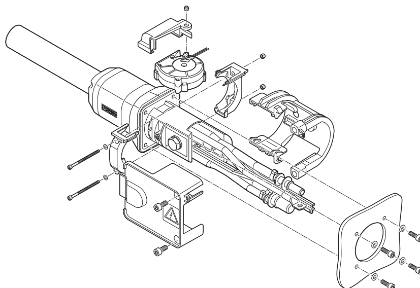
Instructions de montage pour la mise en place de la protection contre les contacts, exemple de la traversée de paroi droite
