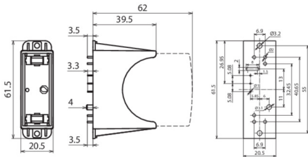
Dimensioni DG PCB I 275 FM
