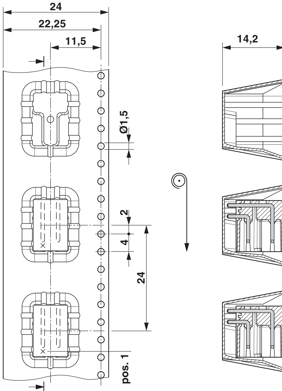
Maßzeichnung
