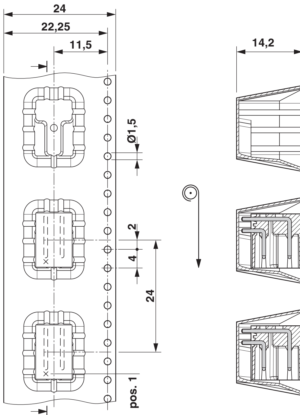
Dessin coté
