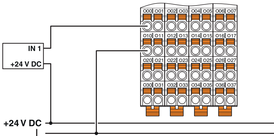
Anschluss von Sensoren beim Einsatz externer Potenzialschienen
