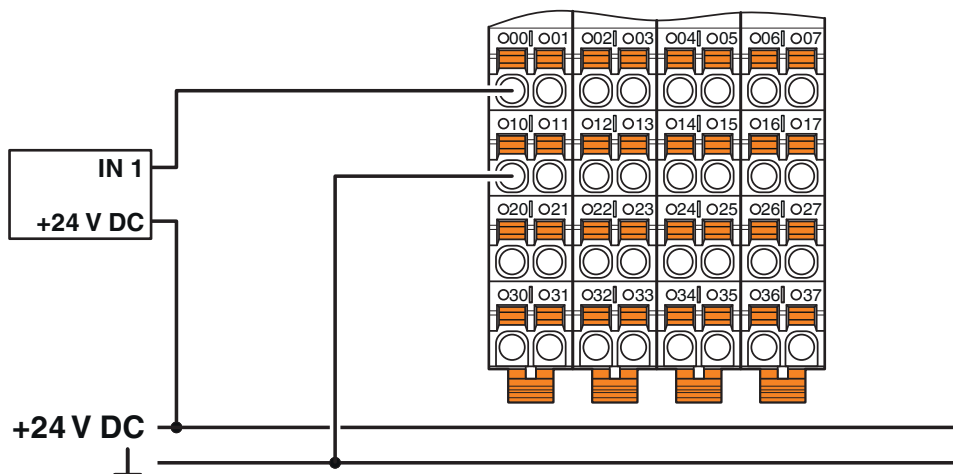
Conexión de sensores para el uso de barras colectoras externas
