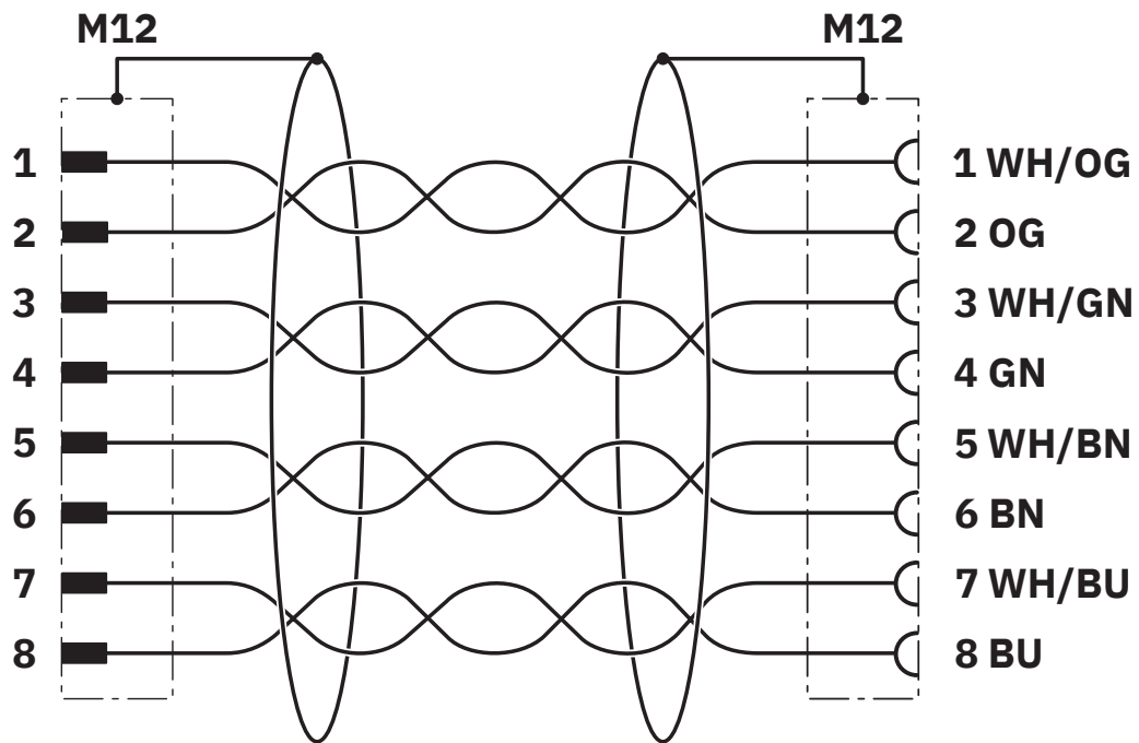
Schaltplan
