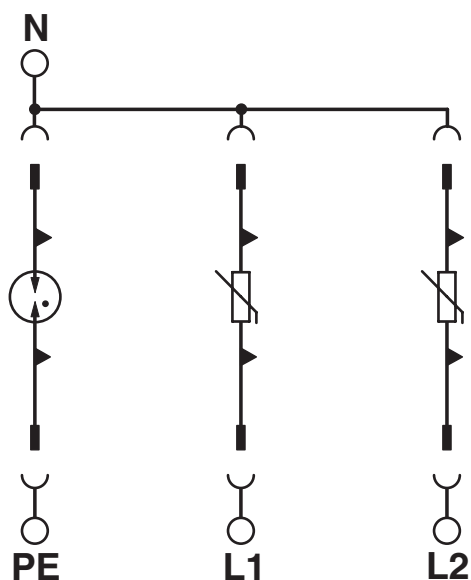
Diagrama eléctrico
