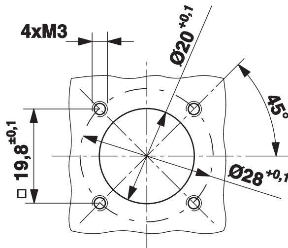
Plano esquemático
