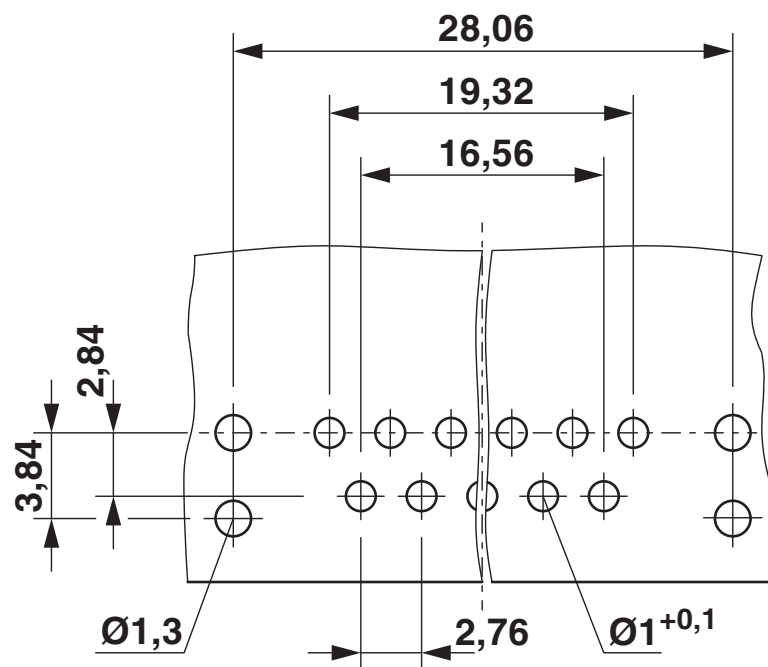
Gabarit perçage / géom. pastille soudage
