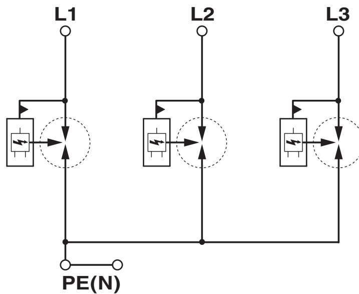
Schaltplan
