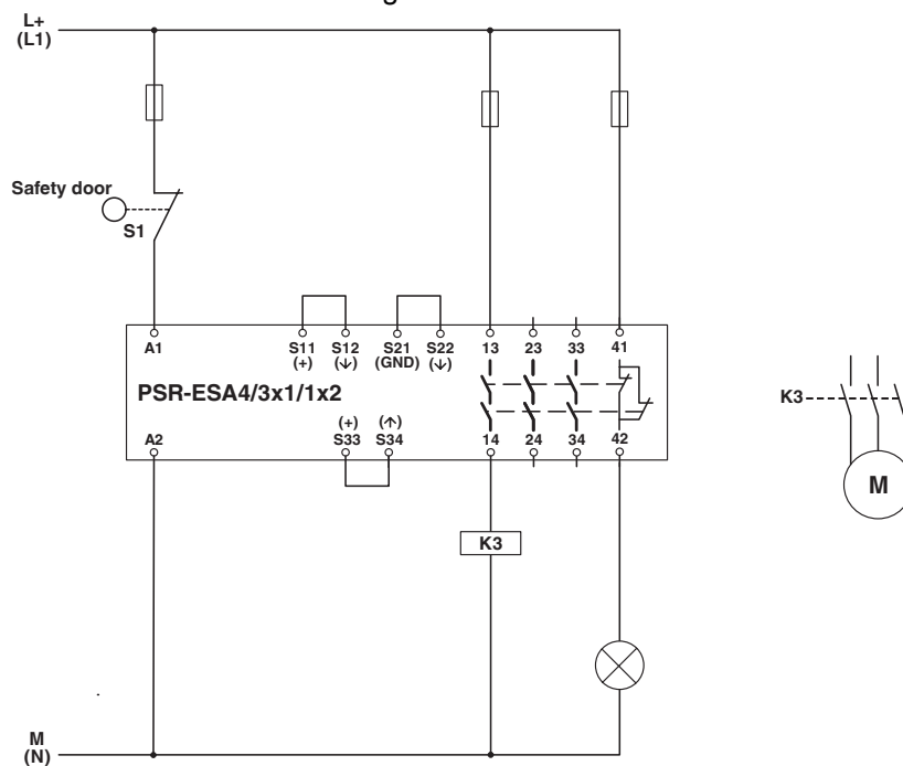
Diagrama eléctrico
