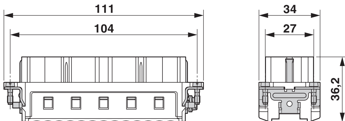
Dessin coté
