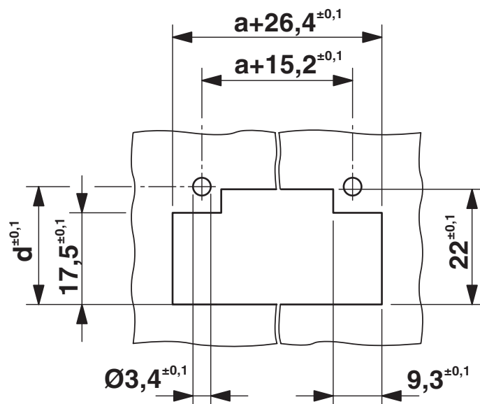
Dessin coté
