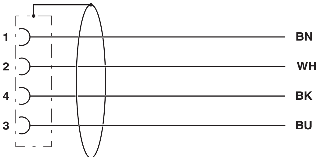
Affectation des contacts du connecteur femelle M8
