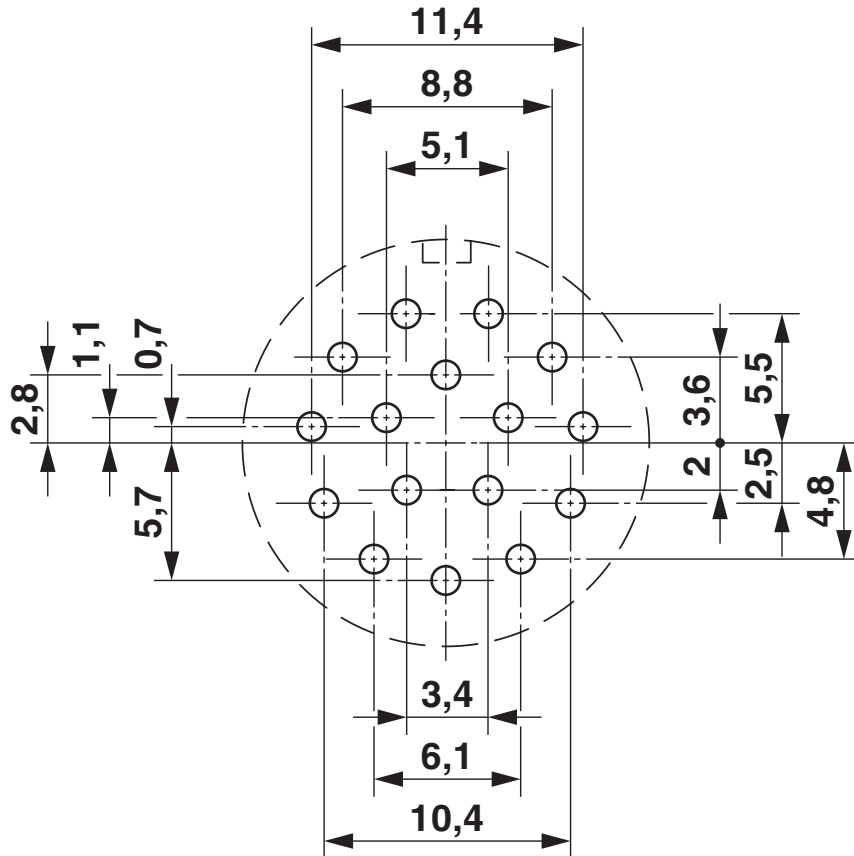
Bohrplan/Lötpadgeometrie
